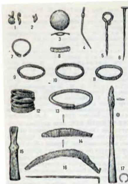
Милоградская культура железного века: 1—13 — бронзовые и железные украшения; 14 и 17 — железный нож и дротик; 15 — железный пластинчатый топорик; 16 — железный серп.
